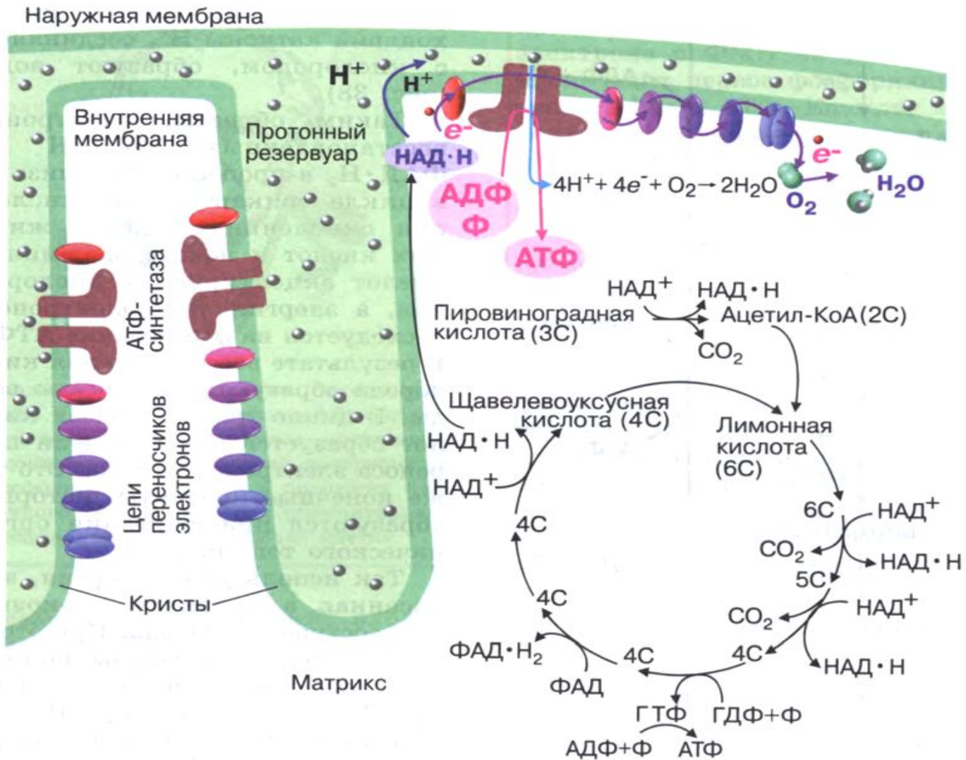
рис. 38. Схема расположения цикла Кребса и цепи переноса электронов в митохондрии
