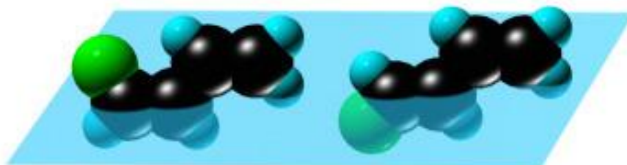
цис-изомер
