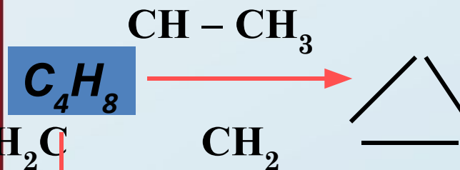
Метилциклопропан
