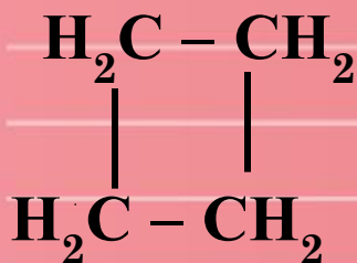
Циклобутан
