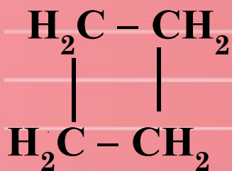
Циклобутан
