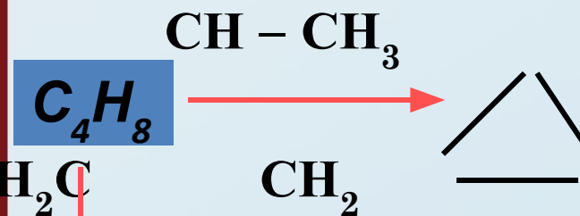
Метилциклопропан
