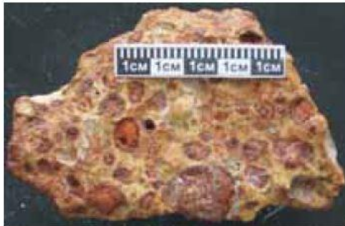
ж-и) бокситы осадочные с бобовой и оолитовой структурой
