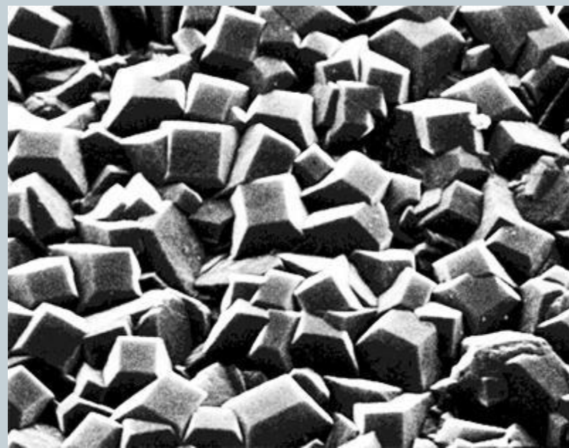
Плавление алмаза.
