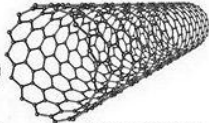
УГЛЕРОДНЫЕ НАНОТРУБКИ
