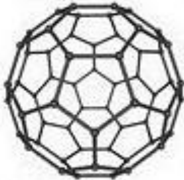
ФУЛЛЕРЕНА
