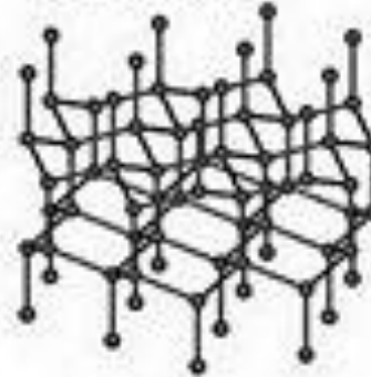
ГРАФИТ
