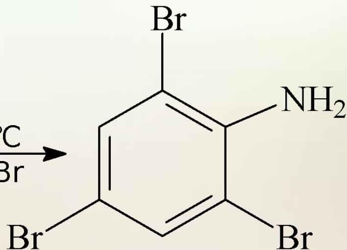
2,4,6-триброманилин
