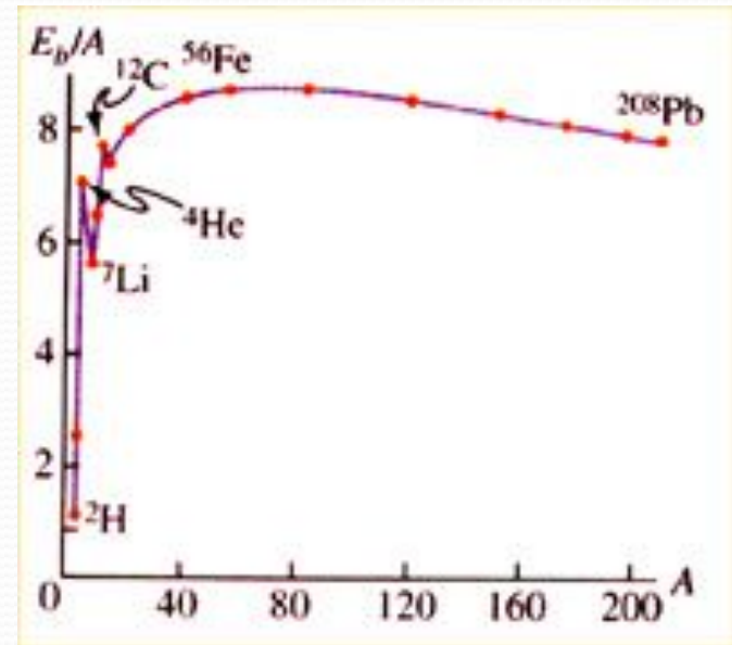
График зависимости удельной энергии связи от массового числа.
