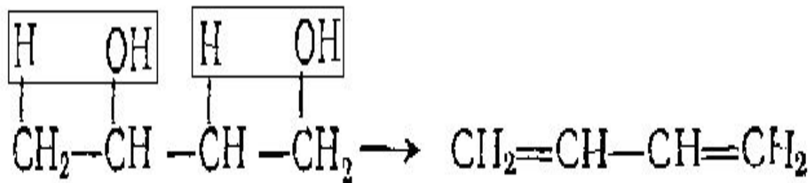
Бутадиен-1,3 (дивинил)
