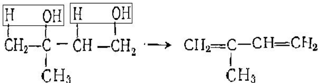
3-МЕТИЛБУТАДИОЛ - 1,3
