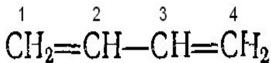
Бутадиен-1,3 (дивинил)
