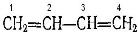
Бутадиен-1,3 (дивинил)
