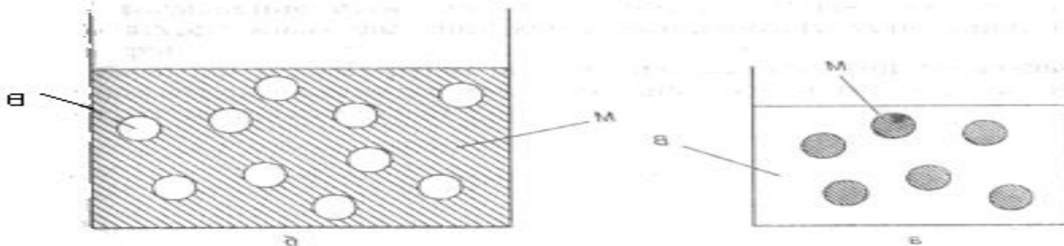
Рис. 1. Типы эмульсий:
