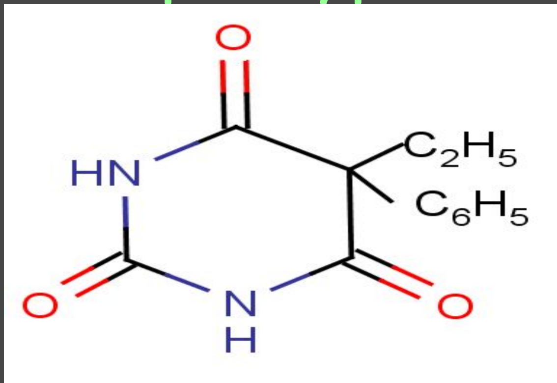
5-этил, 5-фенилбарбитуровая кислота (фенобарбитал)
