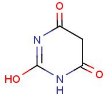
кетоенольная форма
