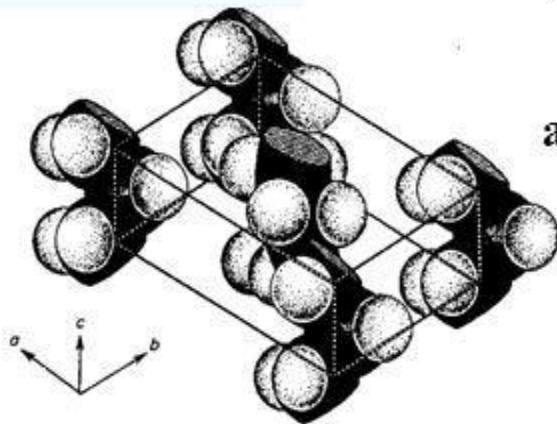
Рис. 10.1. Расположение участков пяти макромолекул полиэтилена в элементарной ячейке кристалла. Размеры ячейки: a = 0,741 \text{ нм}; b = 0,494 \text{ нм}; c = 0,255 \text{ нм}
