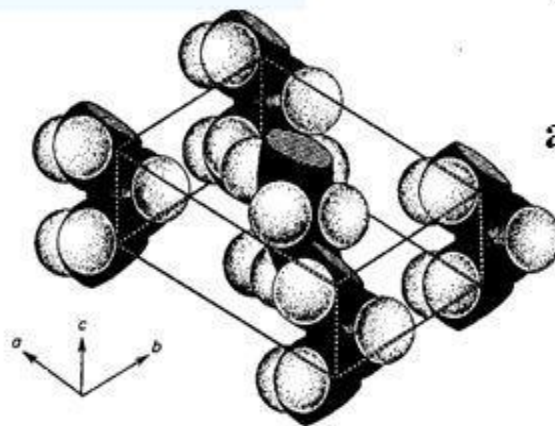
Рис. 10.1. Расположение участков пяти макромолекул полиэтилена в элементарной ячейке кристалла. Размеры ячейки: a = 0,741 нм; b = 0,494 нм; c = 0,255 нм
