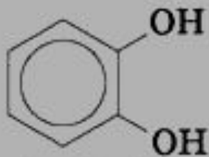
Пірокатехін (1,2-дигідроксibenzen)
