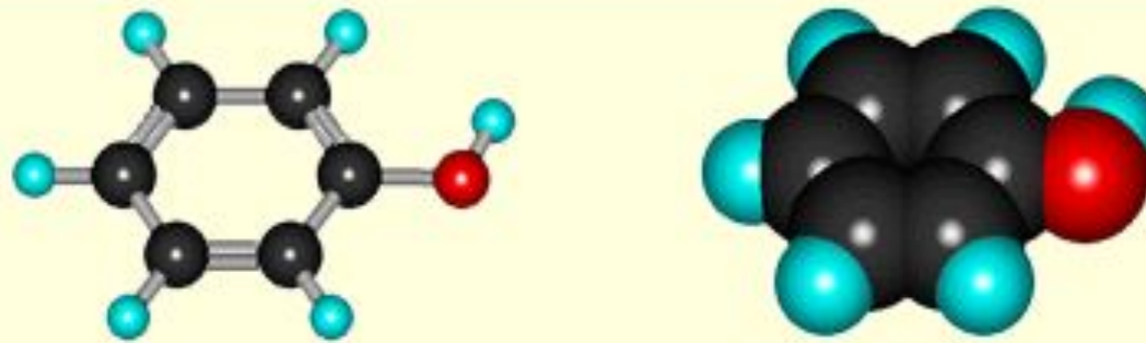
Молекулярные модели
