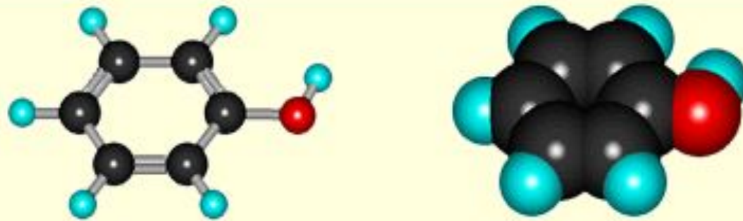
Молекулярные модели
