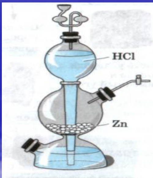
Рис.4 Аппарат Киппа
