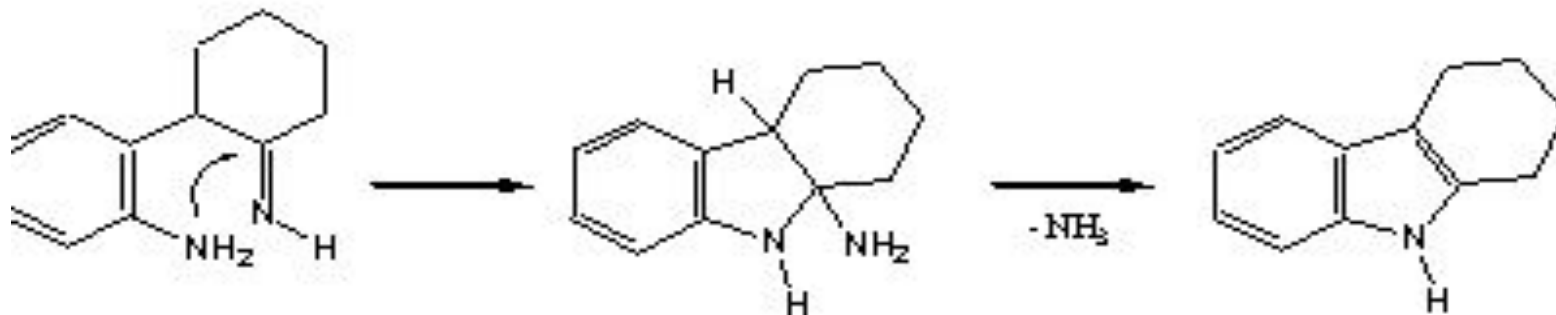
фенилгидразон циклогексанола
