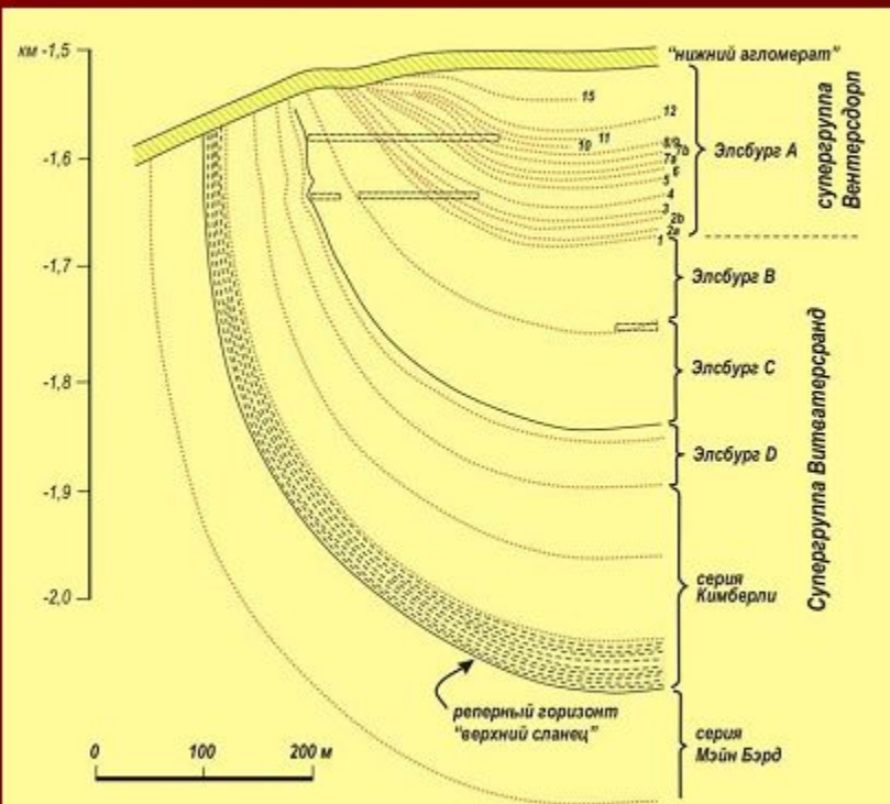
Геологический разрез юго-западного борта бассейна Витватерсранд в районе рудников Лорейн (золоторудное поле Орандж Фри-Стейт) Цветными точечными линиями показаны основные золото-рудные горизонты; пунктиром - горные выработки
