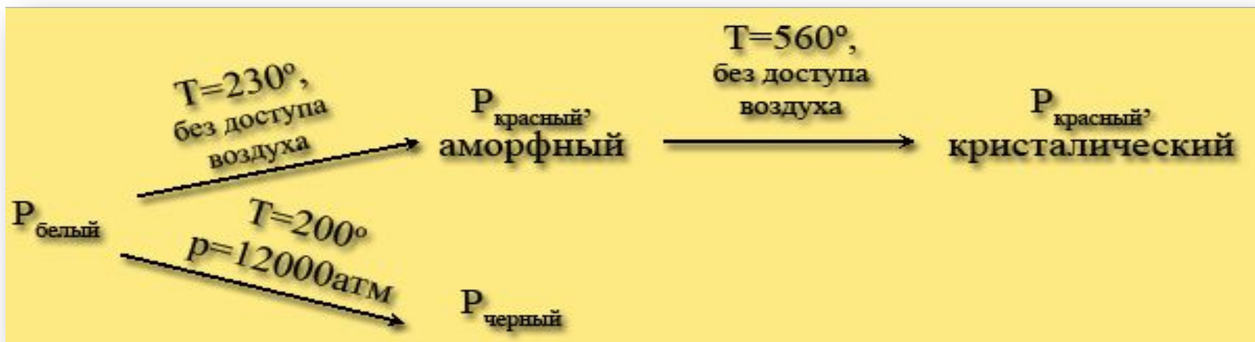
фосфор черный
