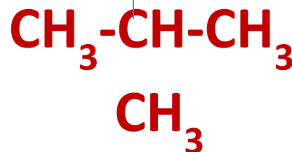
2-метил пропан
