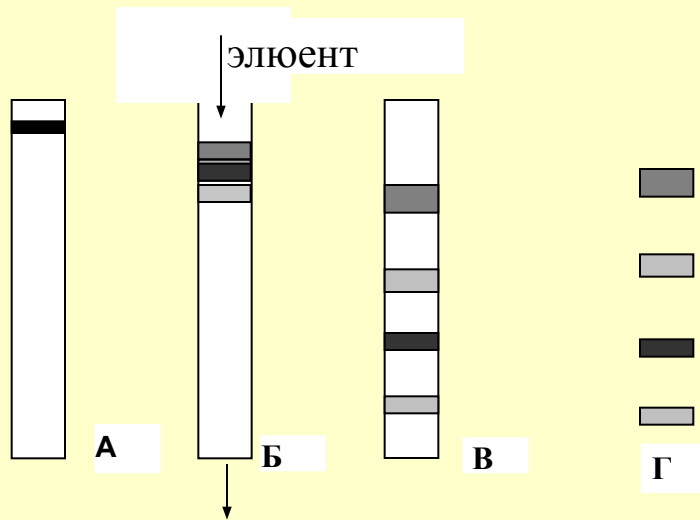
Разделение хлорофилла (1903)
