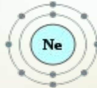
Схема атома неона
