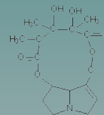
монокроталин
