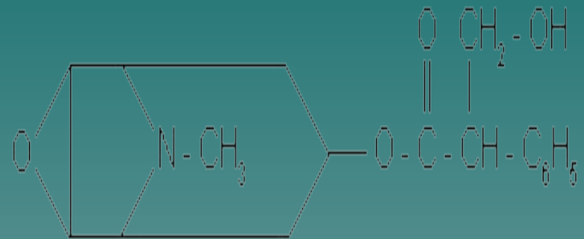
скополамин
