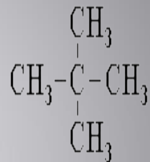
2,2-диметил- пропан
