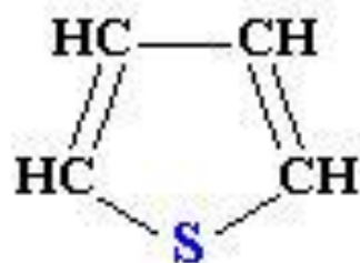
Тиофен
