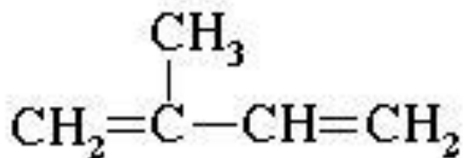
Изопрен
