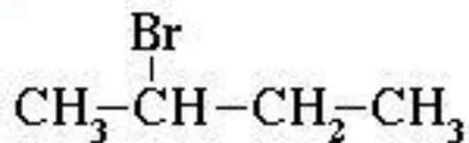
2-Бромбутан
