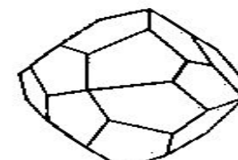
Пентагон-триоктаэдр
