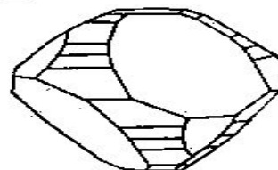
Халькопирит
