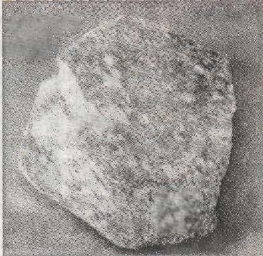
Льдистый кварц
