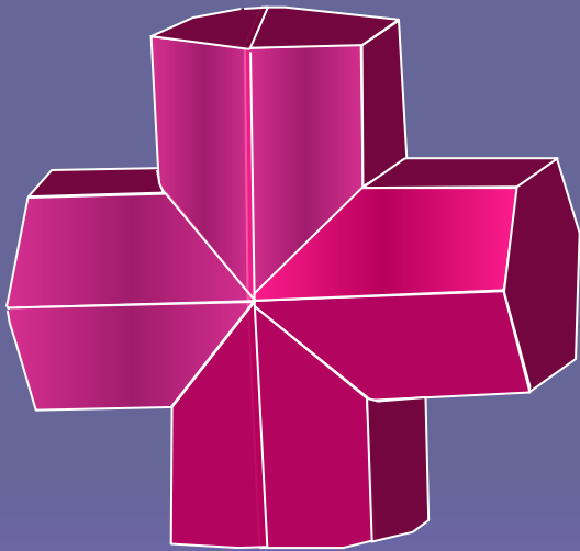
Ставролит
