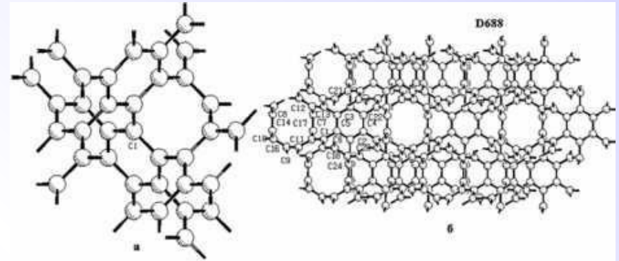
Нанотрубки (модели)
