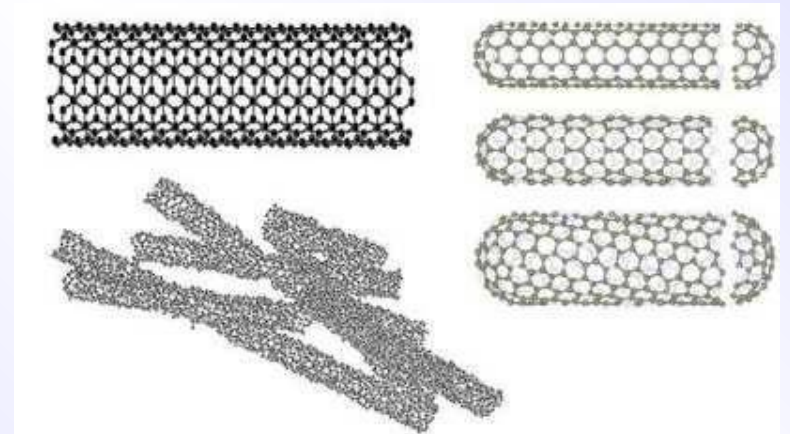
Нанотрубки (модели)
