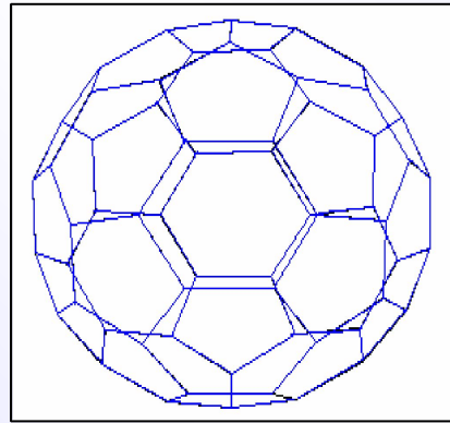
Фуллерен C_{60}
