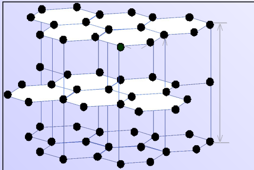
Графит
