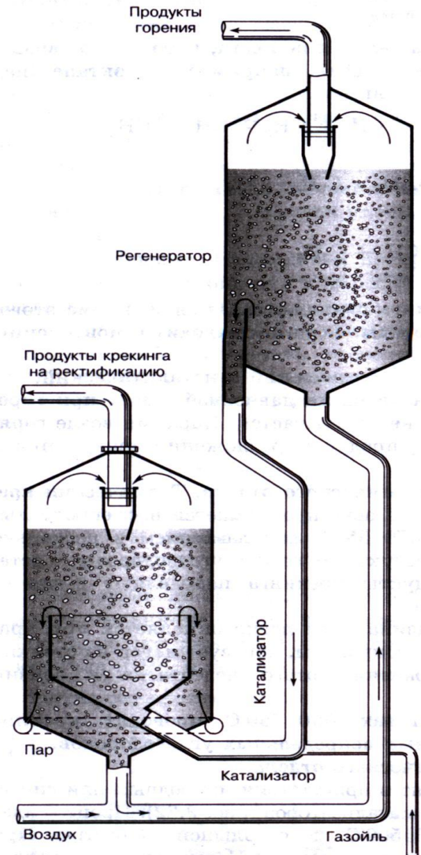
Рис. 2.22. Установа каталітичного крекінгу в "киплячем слоє"
