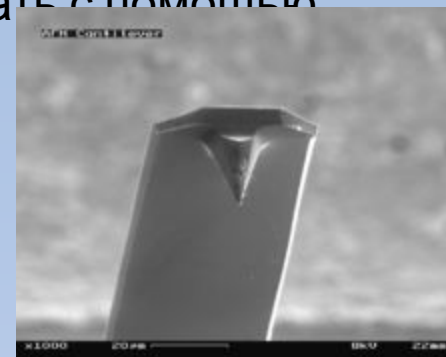
Кантилевер в сканирующем электронном микроскопе (увеличение 1000×)
