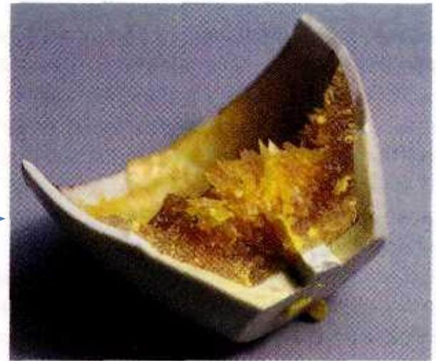
Моноклинная сера
