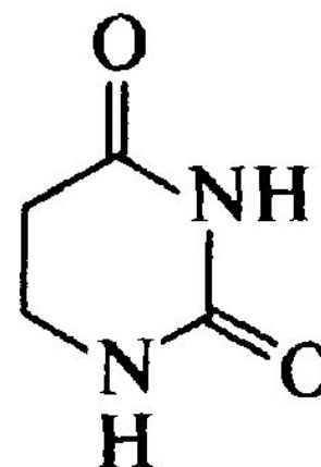
дигидроурацил \text{UH}_2
