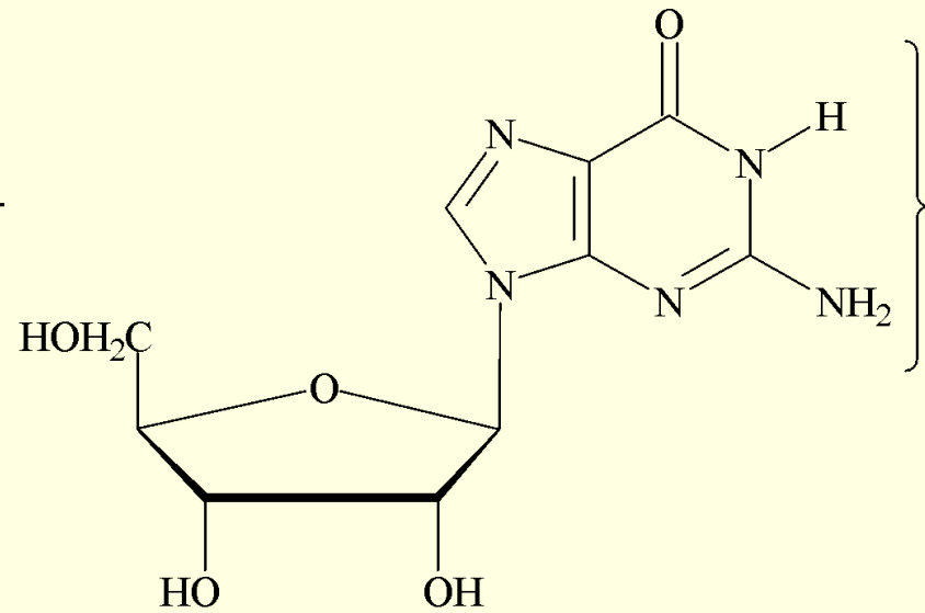
Гуанозин (G)
