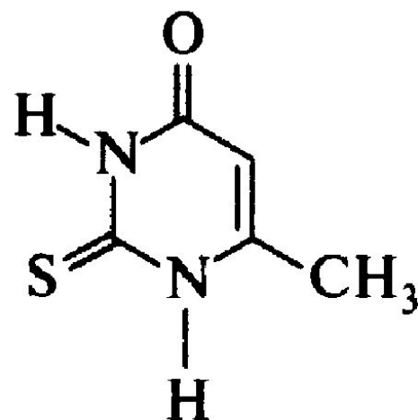
метилтиоурацил
