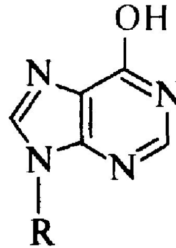
инозин
