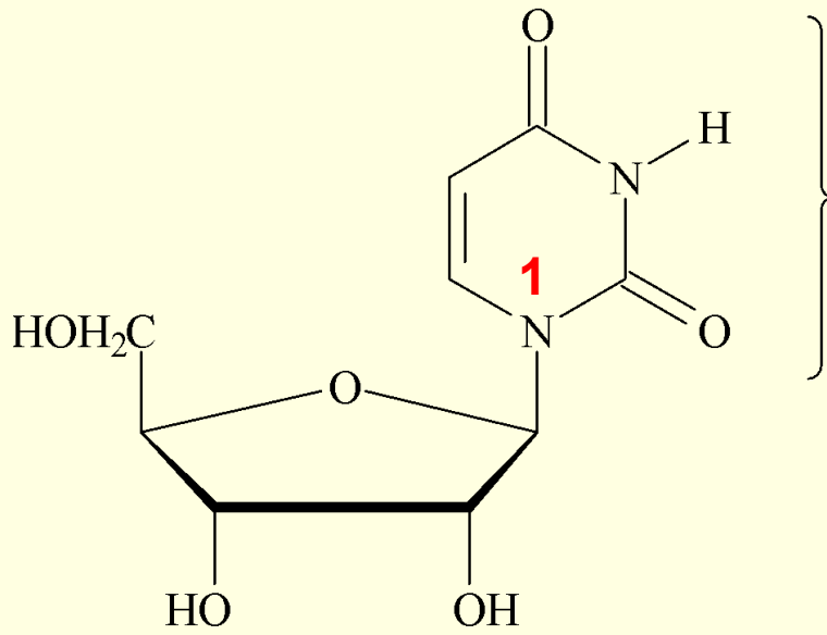
Уридин (U)
