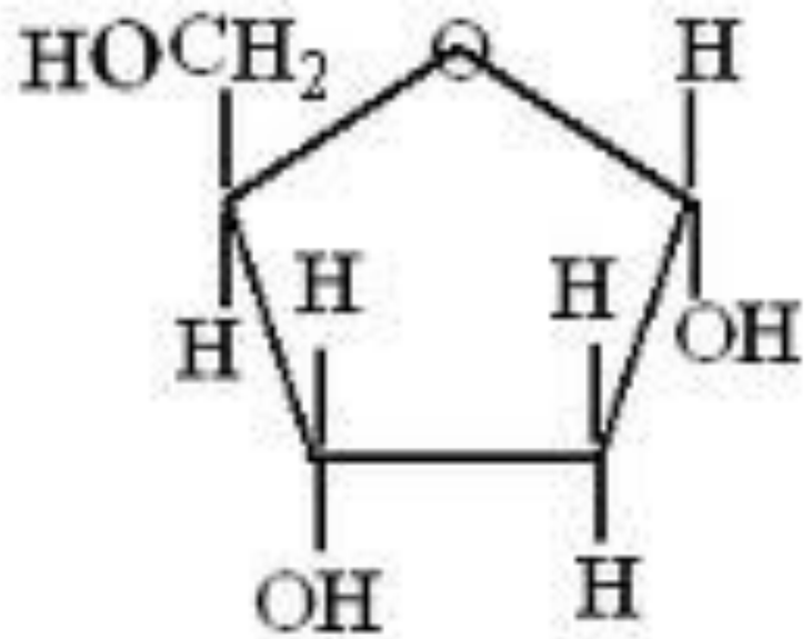
Дезоксирибоза
