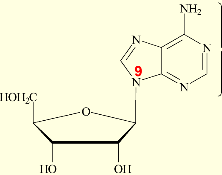
Аденозин (A)
