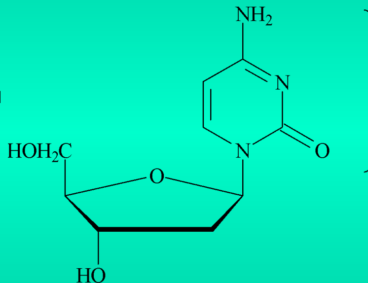
Дезоксицитидин (dC)
