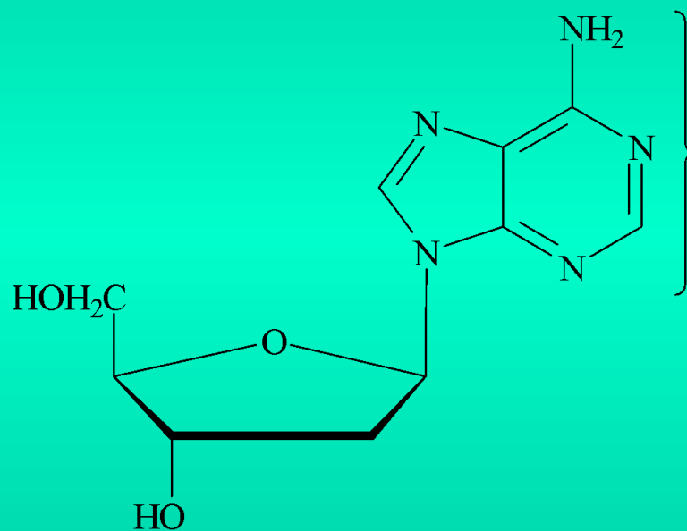
Дезоксиаденозин (dA)
