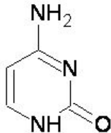
Cytosine
