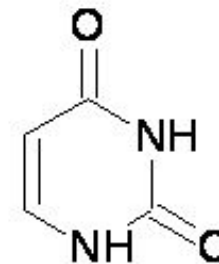
Uracil
