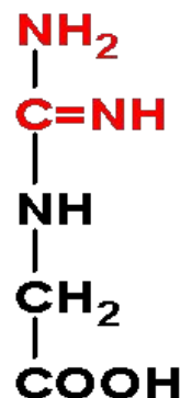
гуанидин- ацетат
