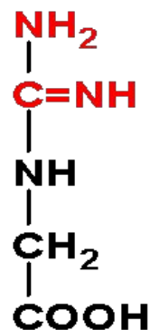
гуанидин- ацетат
