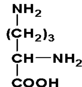
орнитин
