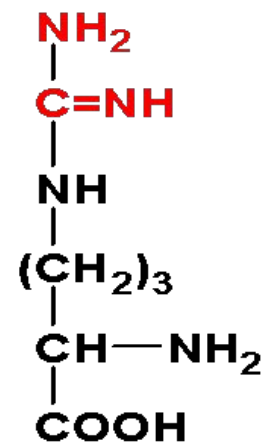
аргинин
