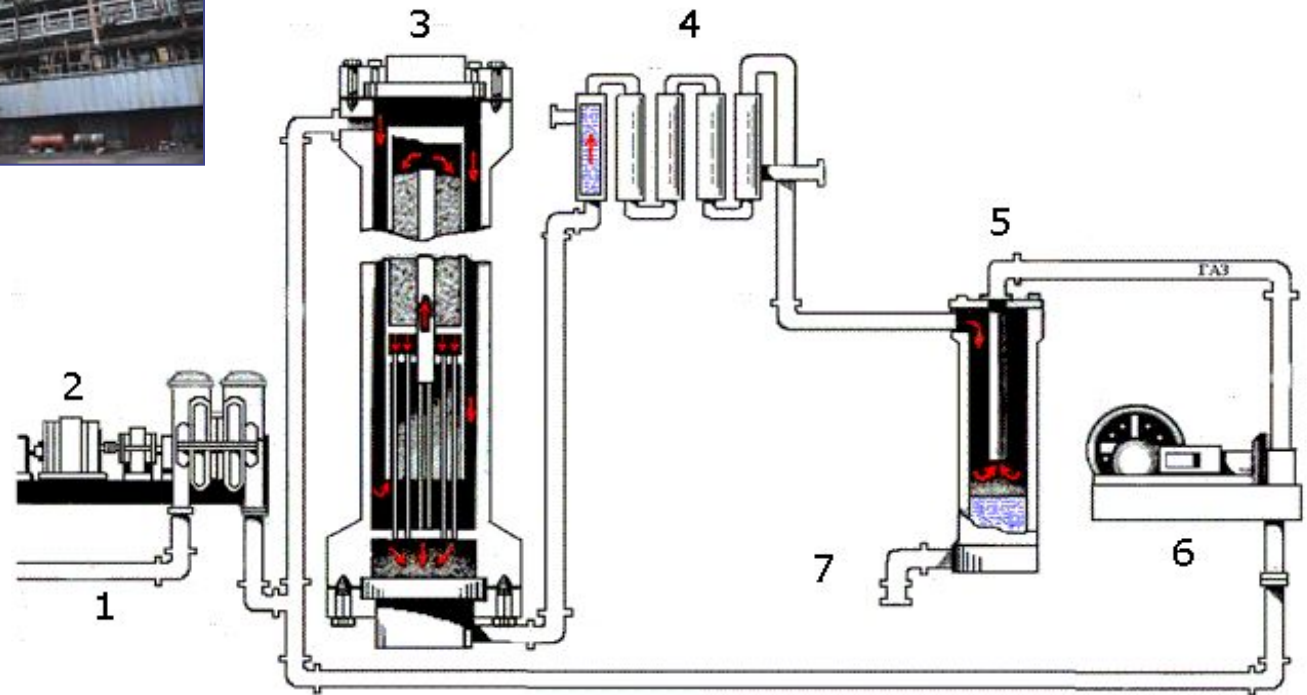
1-азотводородная смесь, 2-турбокомпрессор, 3-колонна синтеза, 4-холодильник, 5-сепаратор, 6-циркуляционный насос, 7-аммиак на склад
