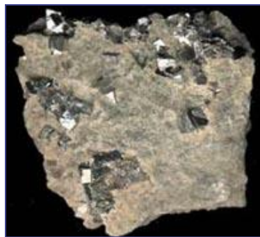
Арсенопирит
