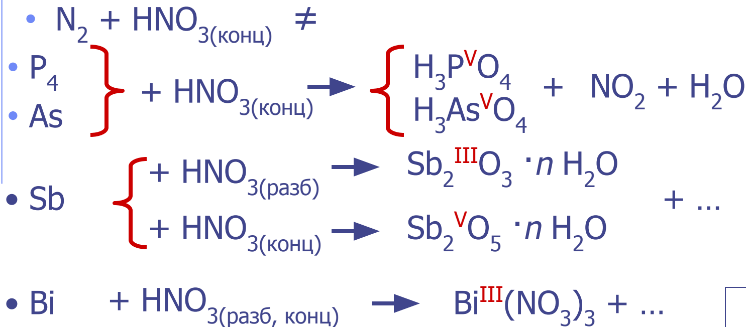
Мышьяк
