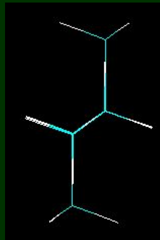
2,3-диметилгексан
