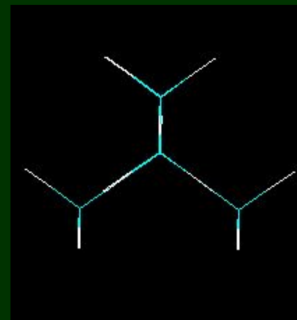
2,2-диметилгексан
