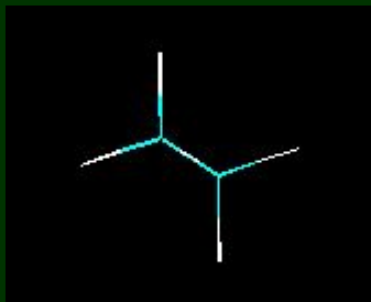
н-октан
