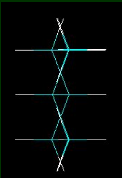
2-метил-3-этилпентан
