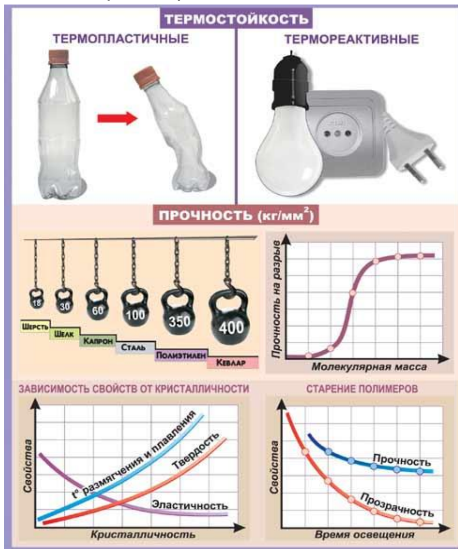
Рис. 6. Свойства полимеров
