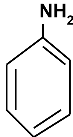
Анилин (аминобензол)
