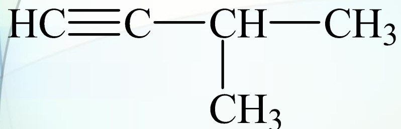
3-метилбутин-1
