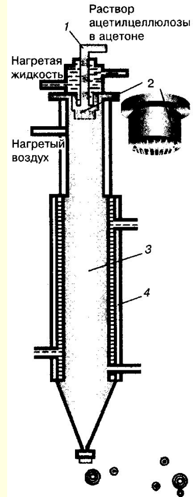
Рис. 29. Схема формования ацетатного волокна: 1 — прядильная головка; 2 — фильтра; 3 — образующиеся волокна; 4 — шакта
