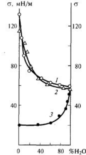
Изотермы поверхностного натяжения воды для солей электролитов в концентрации воды от 0 до 100%
