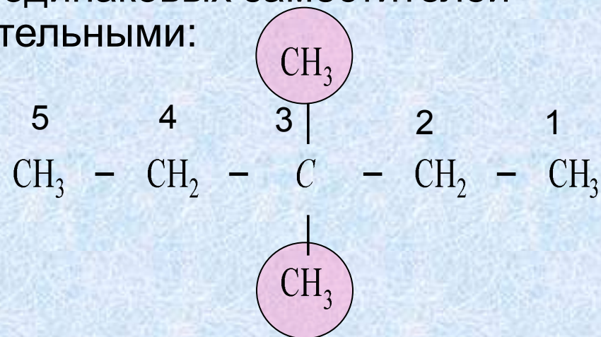
3,3 - Диметилпентан
