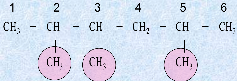
2,3,5 -Триметилгексан
