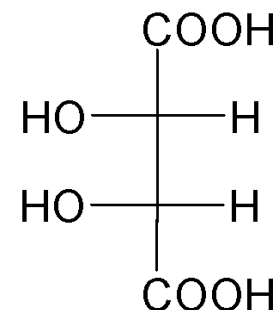
мезовинная кислота
