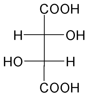
D-винная кислота
