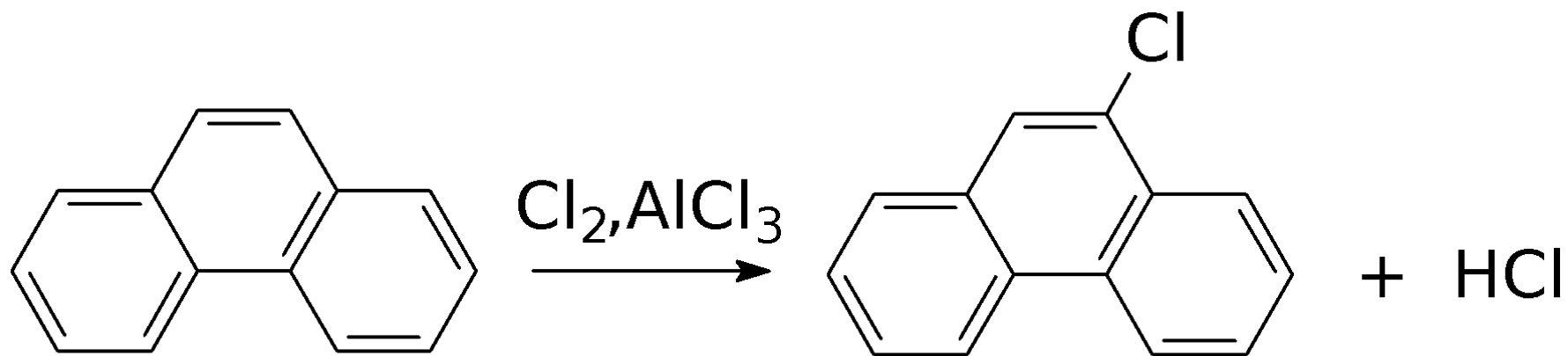
9-Хлорфенантрен
