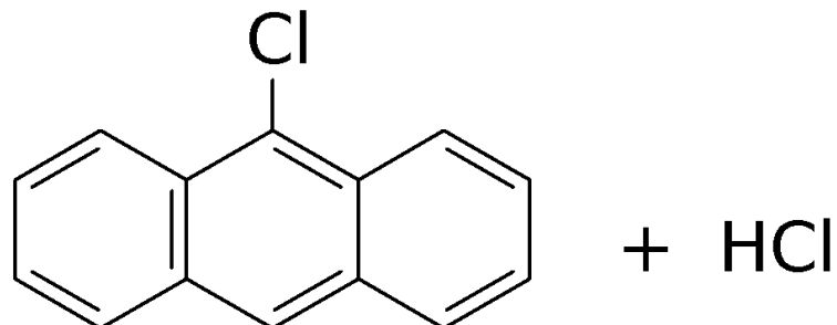
9-Хлорантрацен
