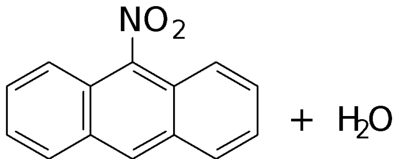
9-Нитроантрацен
