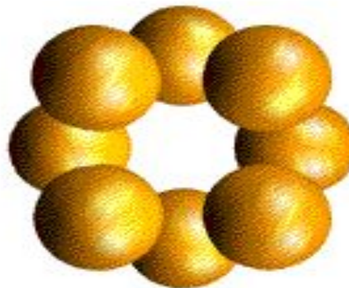
серы S_8
