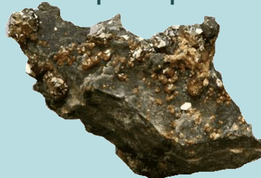
Сфалерит
