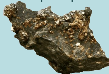
Сфалерит
