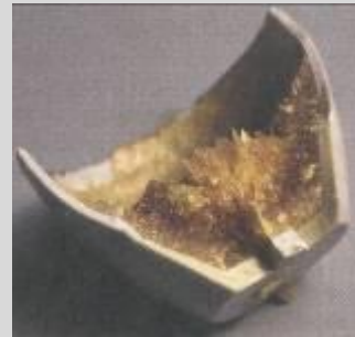
Сера моноклинная
